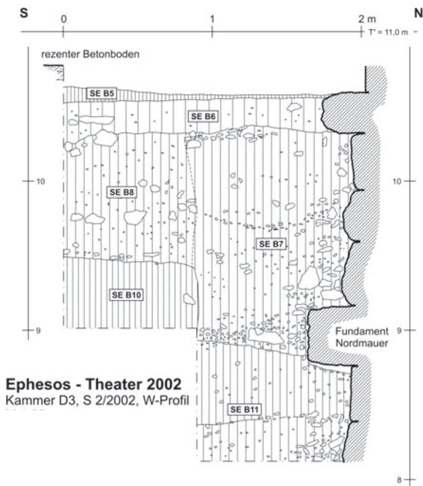
Abb. 30: Kammer D3, S 2/2002, Westprofil
