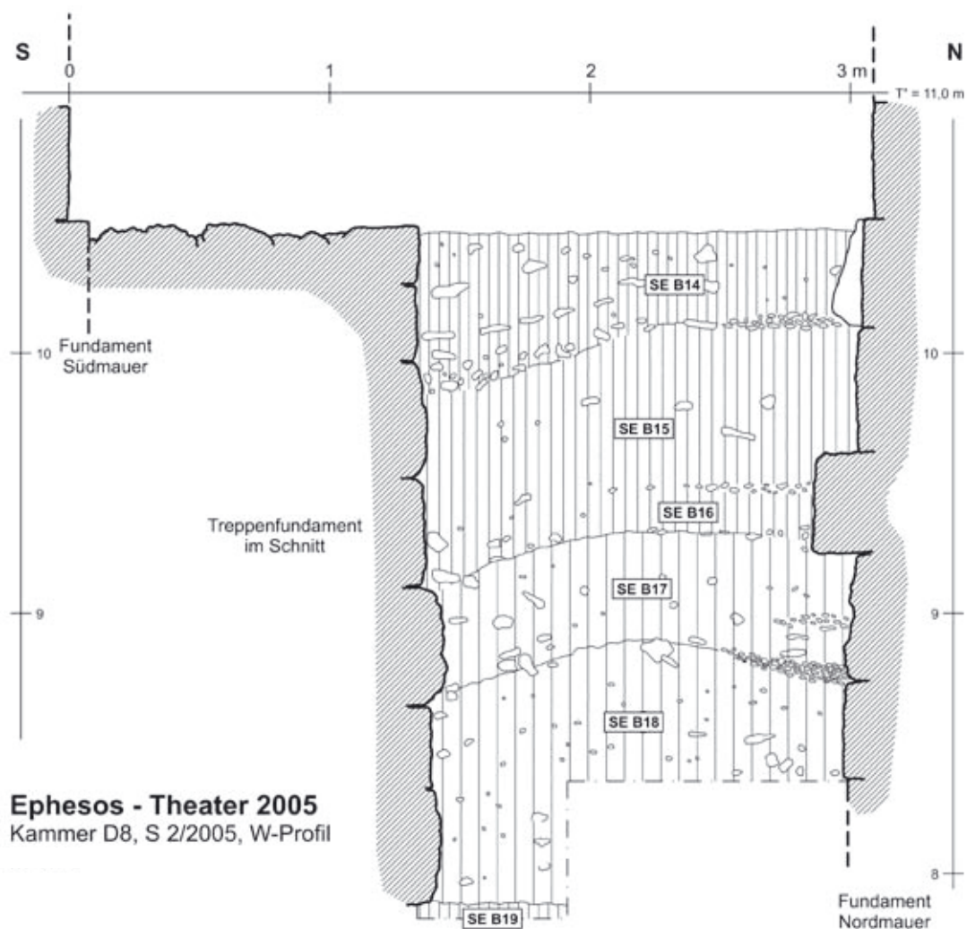
Abb. 33: Kammer D8, S 2/2005, Westprofil
