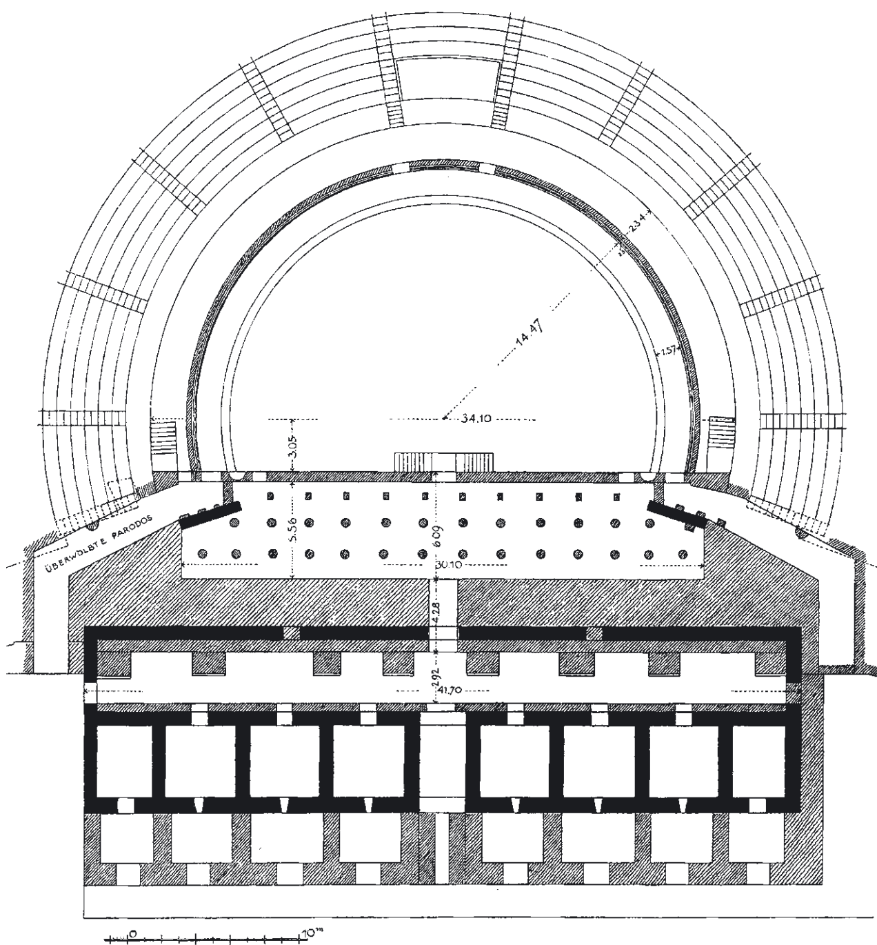
Abb. 20: Grundriss des kaiserzeitlichen Theaters (Rekonstruktion Wilberg 1912)
