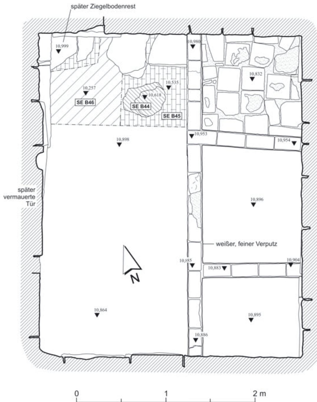
Abb. 47: Kammer E5, zeichnerische Aufnahme
