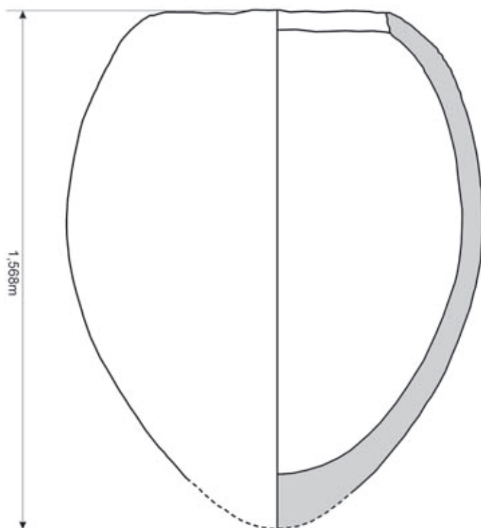
Abb. 45: Kammer E3, Schnitt durch Pithos 1
