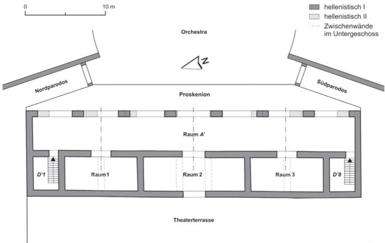
Abb. 19: Grundriss des hellenistischen Obergeschosses (Rekonstruktion Hofbauer 2006)
