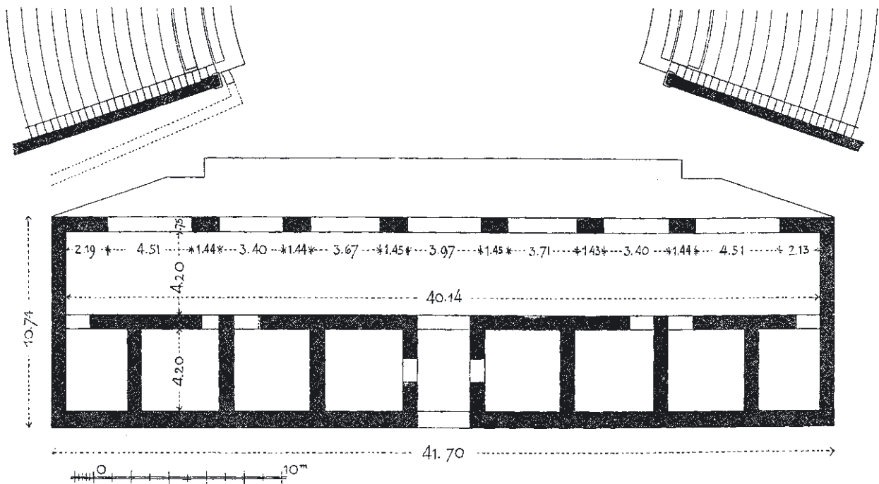
Abb. 18: Grundriss des hellenistischen Obergeschosses (Rekonstruktion Wilberg 1912)
